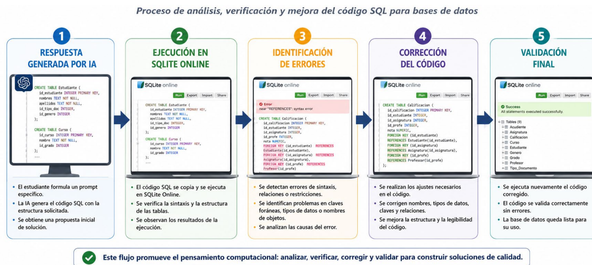
Figura 2 Flujo de validación del código generado por inteligencia artificial
